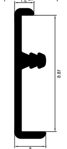
2010 F Çıta Eşit
