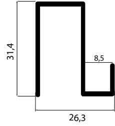
Ara Bağlayıcı (Gizli ara bağlayıcı) (5023)
