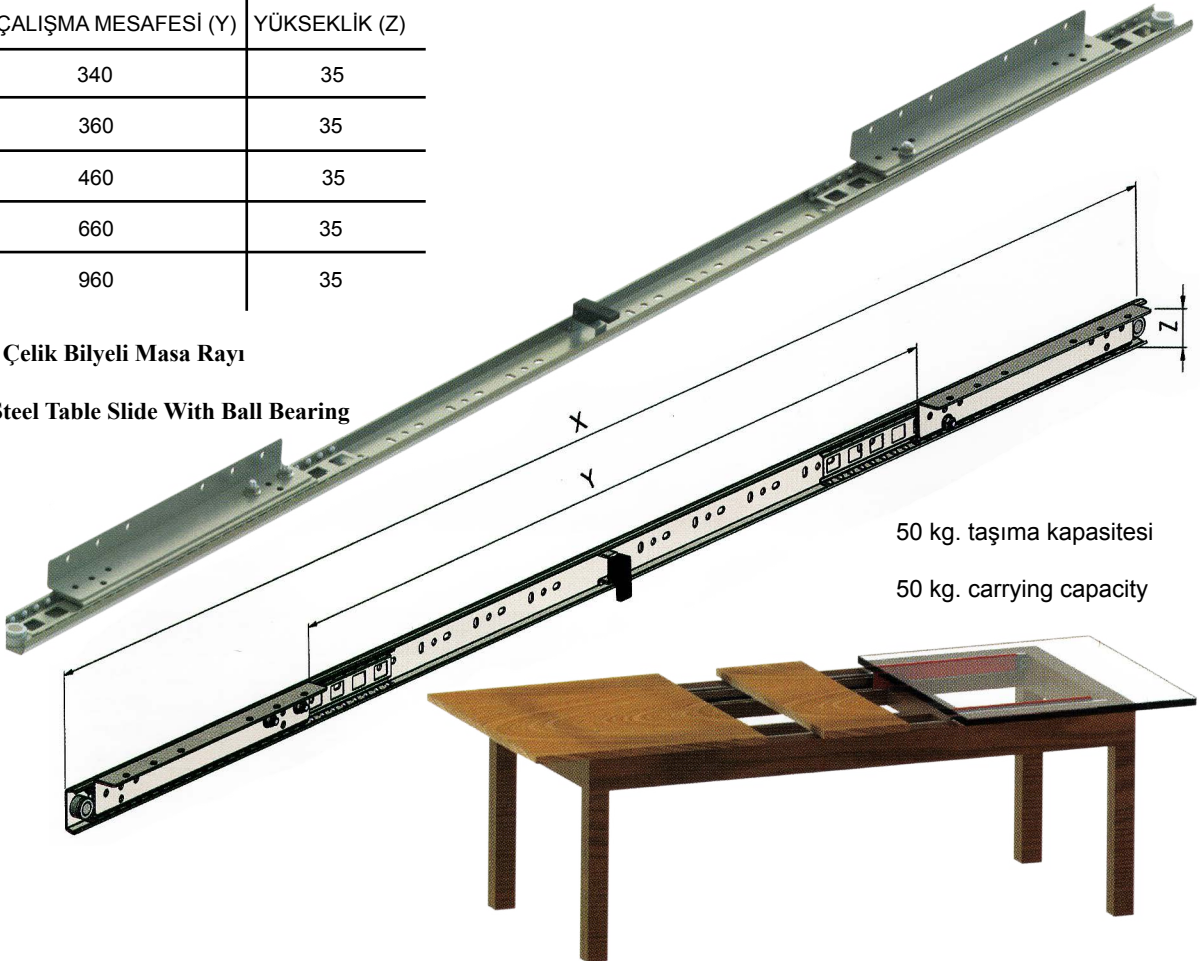
Çift Kanatlı Çelik Bilyeli Masa Rayı
