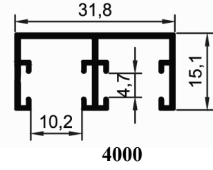
Alt Bağlayıcı
