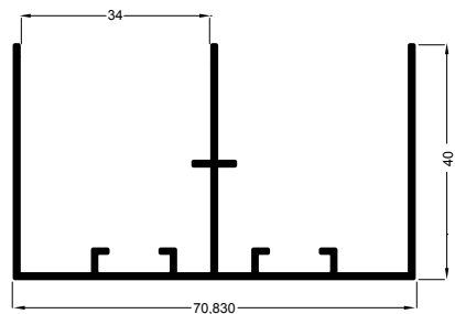
8033 - Üst Ray
