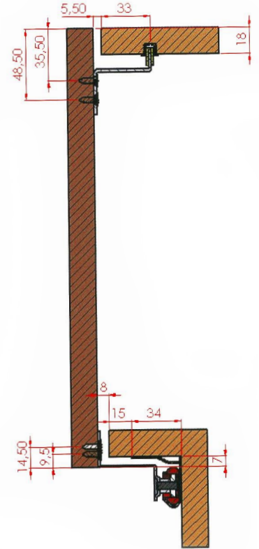
Alt makara Bottom roller
