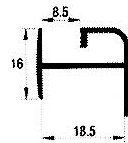
Orta Kayıt Profili
