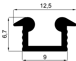
8010 - Alt Ray
