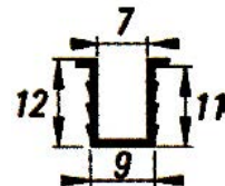
PVC Alt Klavuz
