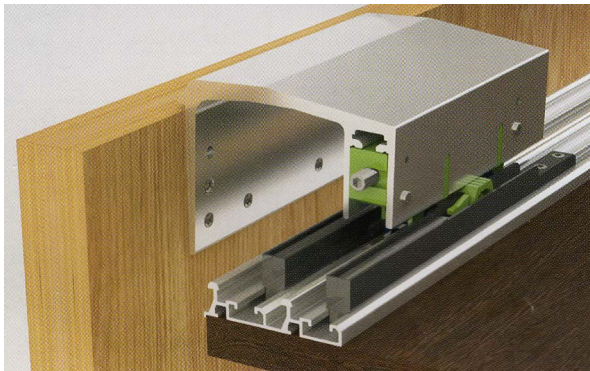
Alüminyum Üst Ray
