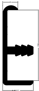
2010 F Çıta Geniş
